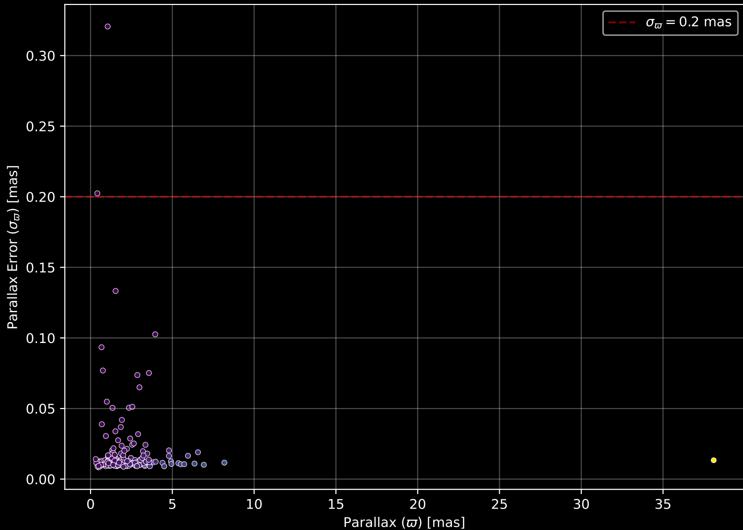
GALAH DR4 Field: [7189] Parallax Quality (n= 202)
