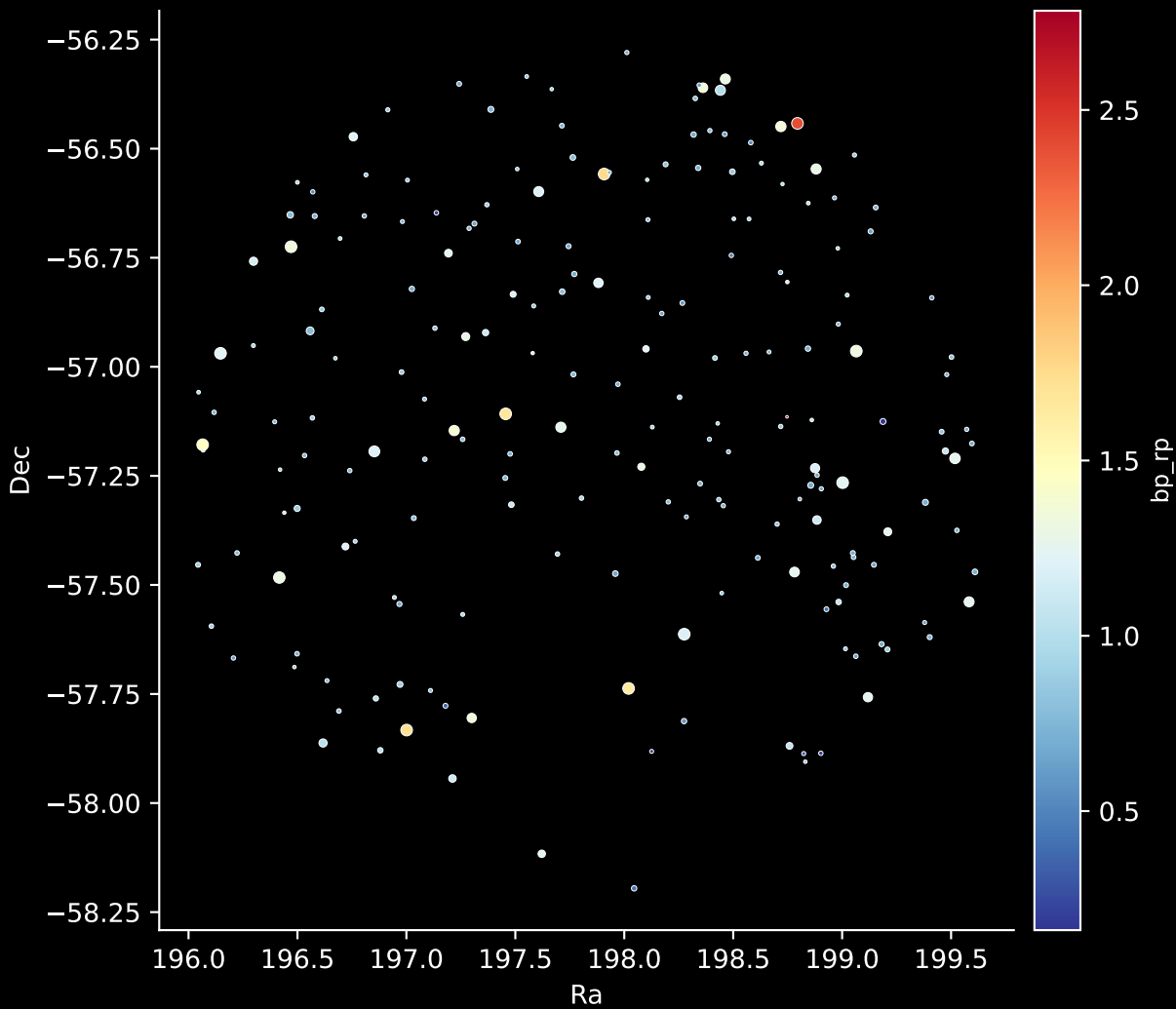
GALAH DR4 Field: [7189] Stars: 202
