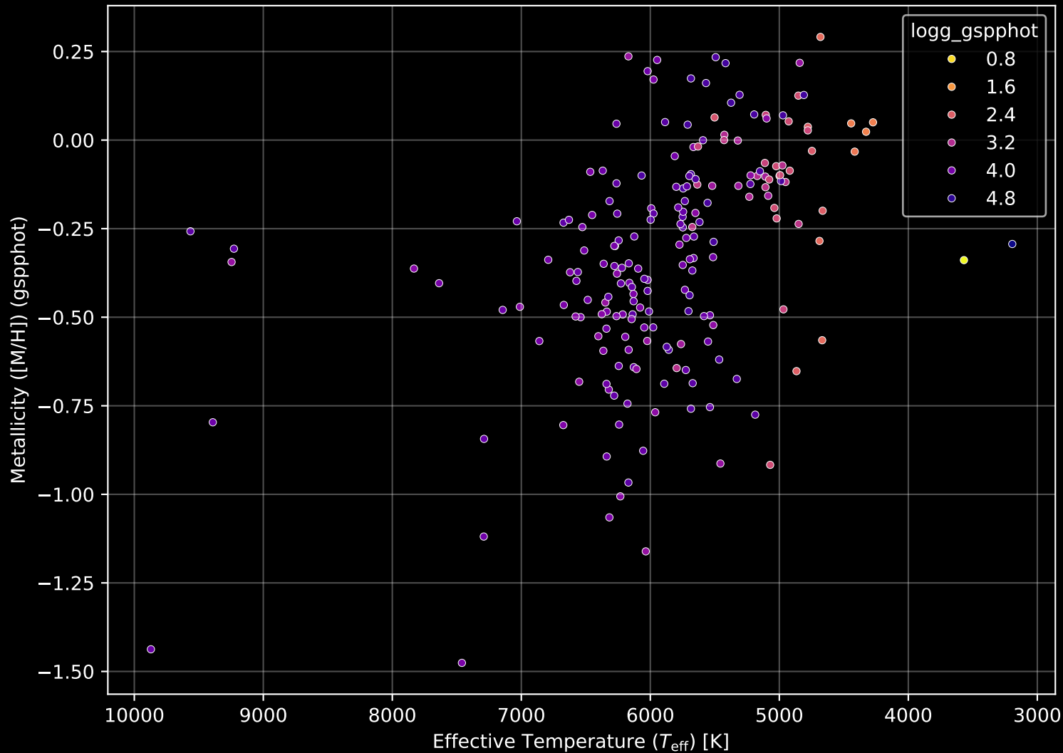
GALAH DR4 Field: [7189] Stellar Population Parameters (n= 202)
